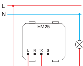
(1) δισύρματη σύνδεση
