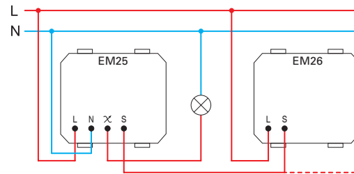
(2) τρισύρματη σύνδεση
