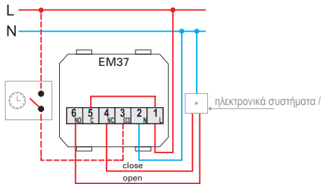
μηχανοκίνητη οδήγηση (περιορισμένη χρήση με ενδοδαπέδια θέρμανση) /
