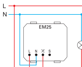
(2) τρिसύρματη σύνδεση
