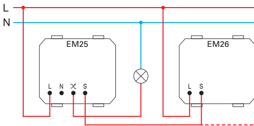
(1) δισύρματη σύνδεση
