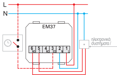
λέβητας, κυκλοφορητής, καυστήρας (T1/T2 εισόδου ελέγχου) /
